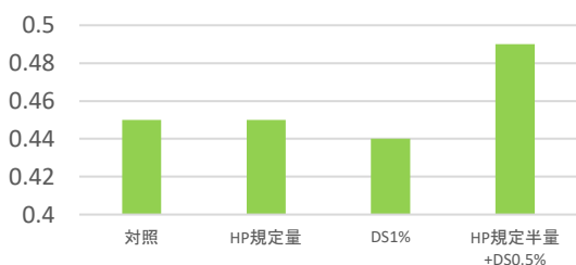
陰圧解除後の瞬時の戻り/最大吸引高 塗布後15分
